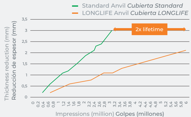
Anvil lifetime comparative chart Comparativa tiempo de vida
