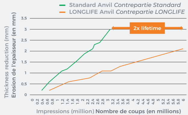
Anvil lifetime comparative chart Comparatif durée d'utilisation
